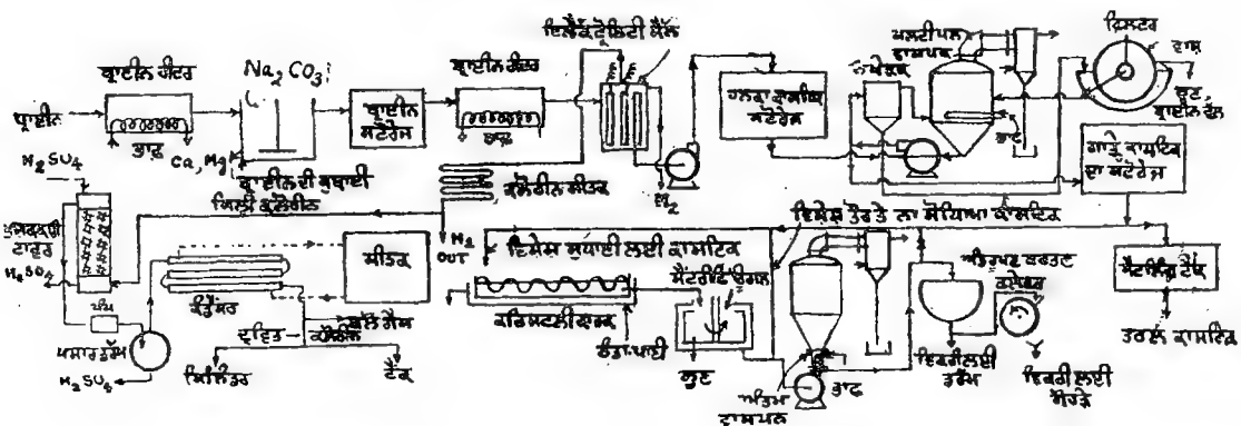
ਚਿਤਰ 2. ਬਿਜਲ-ਅਪਘਟਨੀ ਕਾਸਟਿਕ ਸੋਡਾ ਅਤੇ ਕਲੋਰੀਨ
