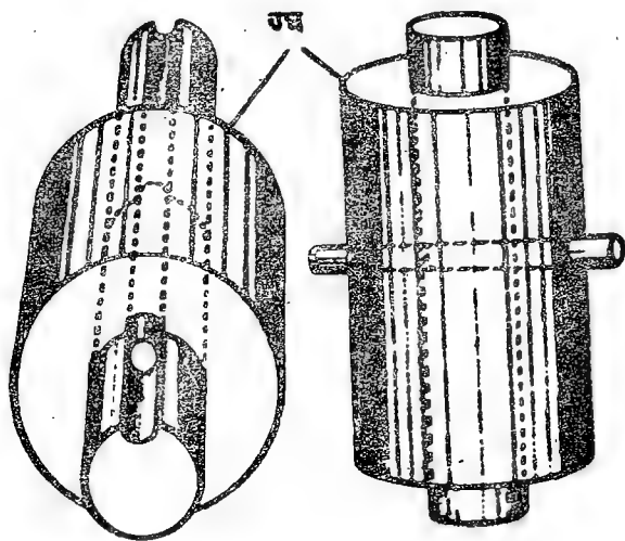
ਚਿਤਰ 2. ਪਿਨ-ਕੁੰਜੀ ਜੋੜਨਾ; (ੳ) ਸ਼ਾਫਟ ਦੀ ਦਿਸ਼ਾ ਵਿਚ; (ਅ) ਸ਼ਾਫਟ ਵਿਚੋਂ ਦੀ।
