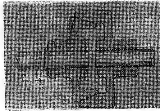
ਚਿੱਤਰ 2. ਸਪਰਿੰਗ ਲੌਡਿਡ ਕੌਨ ਕਲੱਚ
