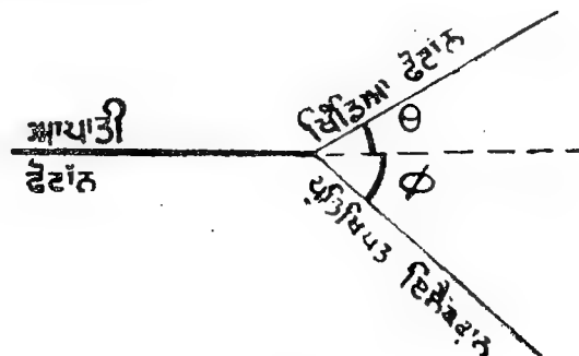
ਕਾਂਪਟਨ ਪ੍ਰਭਾਵ
